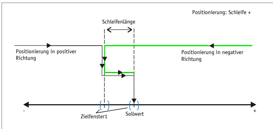
Abb. 4: Positionierung Schleife+
